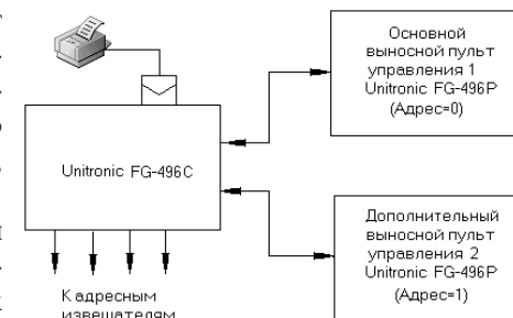
Рис. 4. Схема подключения контроллера к двум выносными пультами управления
