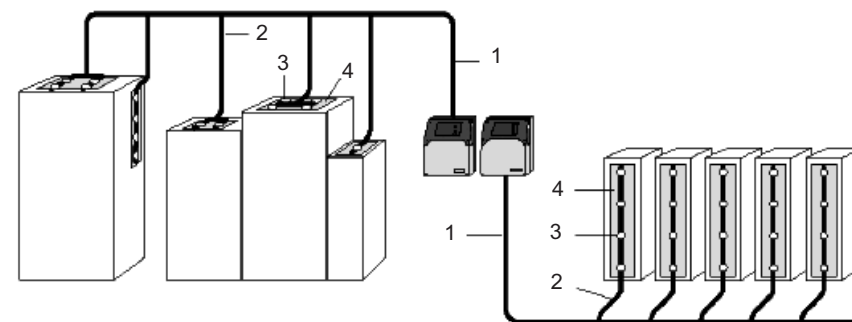
Пример защиты оборудования: 1 — главная труба; 2 — трубы ответвления; 3 — насадки; 4 — вентиляционные отверстия.
